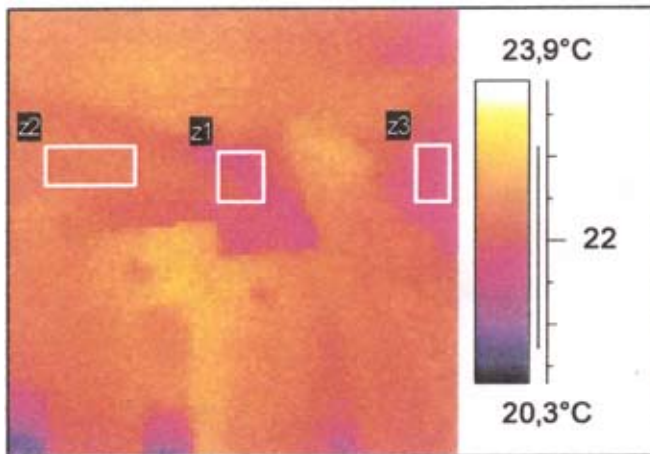
Apšiltinus EKOVATA
