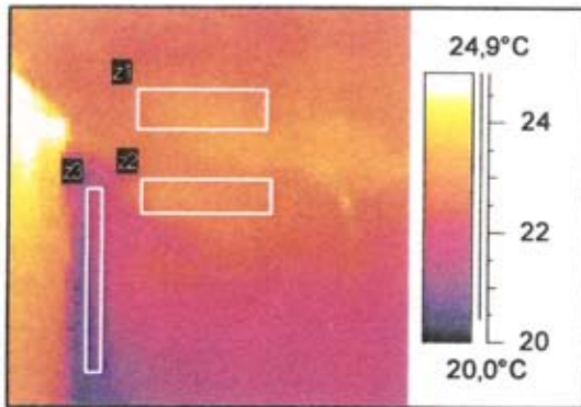
Apšiltinus EKOVATA
